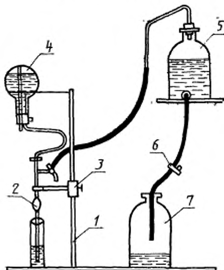
1 — штатив, 2 — пипетка вместимостью 25 \text{ см}^3 , 3 — упор, 4 — колба для промывания пипетки, 5 — аспиратор; 6 — зажим, 7 — водослив
