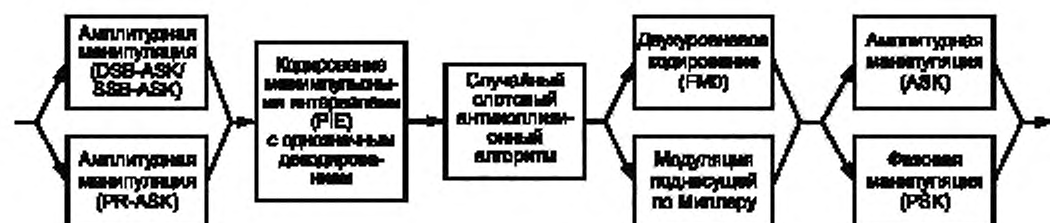
Рисунок 7 — Структура радиочастотной метки типа C
