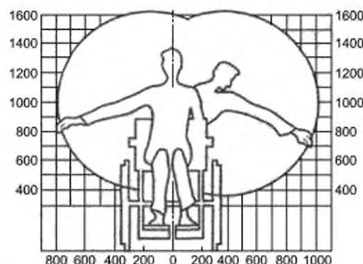
Зоны досягаемости для инвалидов в кресле-коляске
