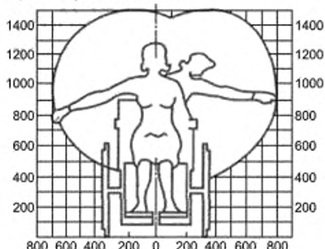
Зоны досягаемости для инвалидов в кресле-коляске
