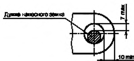
Рисунок 5 — Проушина под навесной замок
