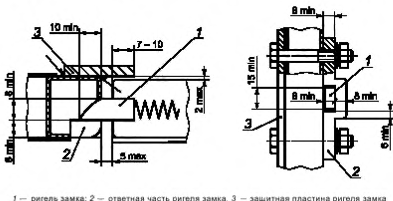
Рисунок 3 — Варианты установки замков дверей отсека для задержанных
