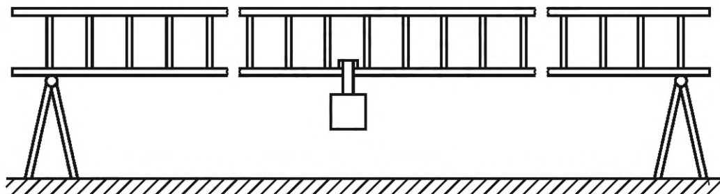
Рисунок 2 — Схема подвески контрольного груза
