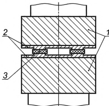
1 — опорные плиты; 2 — сменные пластины с контактными выступами; 3 — образец материала ТРГ
