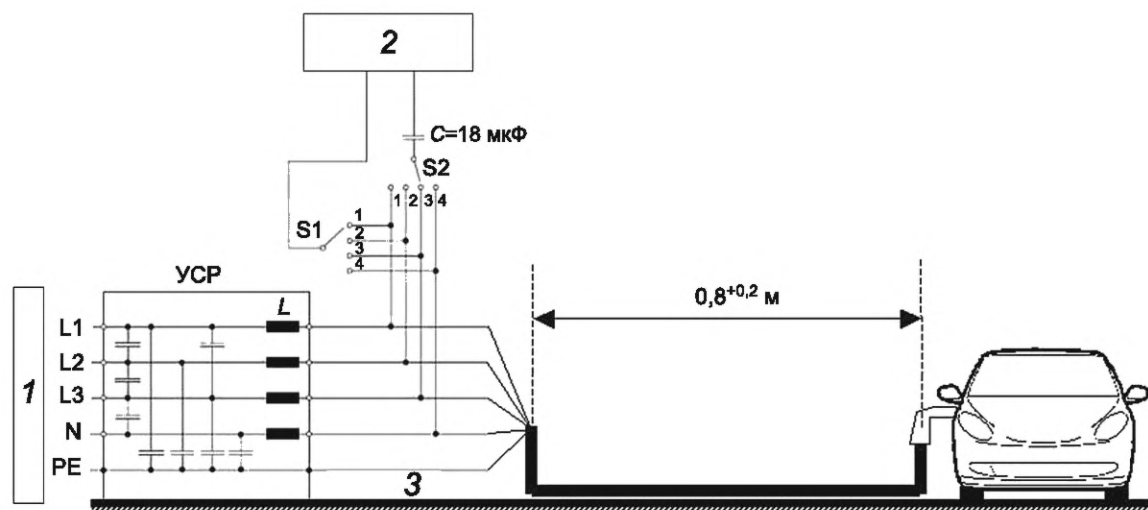
Рисунок 3 — ЭМ в конфигурации «ПСХЭЭ в режиме зарядки, подключенная к электрической сети» — сопряжение каждой фазы и земли в однофазной линии переменного напряжения и линии постоянного напряжения
