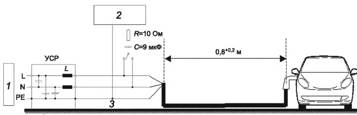
Рисунок 2 — ЭМ в конфигурации «ПСХЭЭ в режиме зарядки, подключенная к электрической сети» — сопряжение однофазной линии переменного напряжения и линии постоянного напряжения
