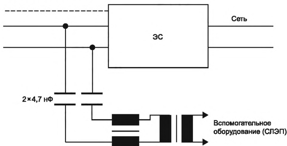
Рисунок А.9 — Пример схемы для испытаний СЛЭП на помехоустойчивость в силовых линиях переменного и постоянного напряжения
