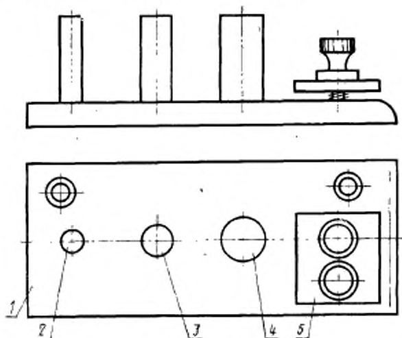
1 — плита; 2, 3, 4 — стержни; 5 — пластина для закрепления образцов
