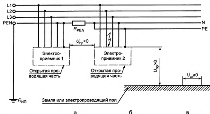
Рисунок В.8 — Сеть TN-C-S с однофазным замыканием на корпус после точки разделения PEN-проводника на N- и PE-проводники
