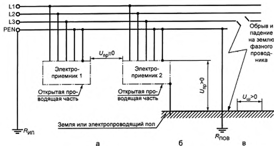
Рисунок В.4 — Сеть TN-C с замыканием на землю, например с оборванным и упавшим на землю фазным проводом
