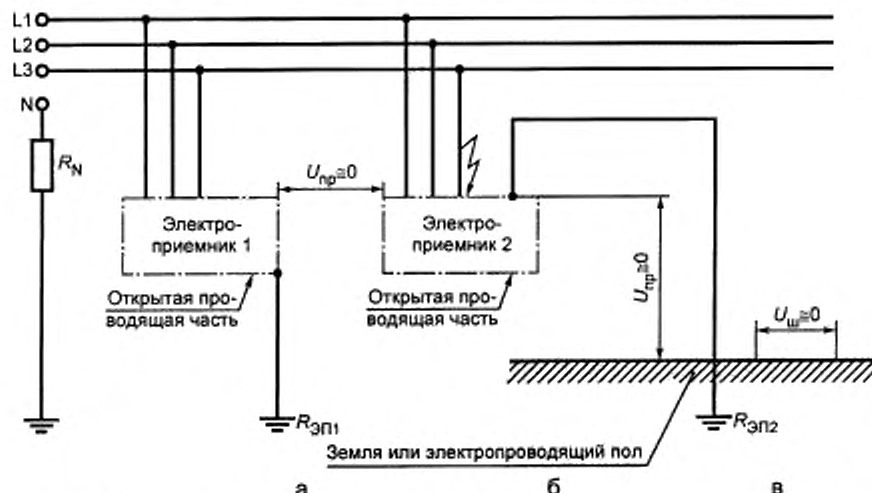
Рисунок В.12 — Сеть IT с заземлением нейтрали источника питания через сопротивление с однофазным замыканием на корпус
