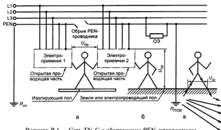
Рисунок В.1 — Сеть TN-C с оборванным PEN-проводником. Уравнивание и выравнивание потенциалов отсутствуют
