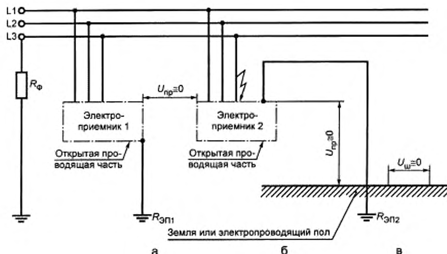
Рисунок В.13 — Сеть IT с заземлением фазы источника питания через сопротивление с однофазным замыканием на корпус
