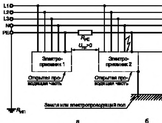
Рисунок В.6 — Сеть TN-S с однофазным замыканием на корпус
