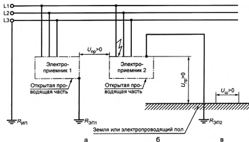
Рисунок В.11 — Сеть ТТ без нулевого рабочего проводника с однофазным замыканием на корпус
