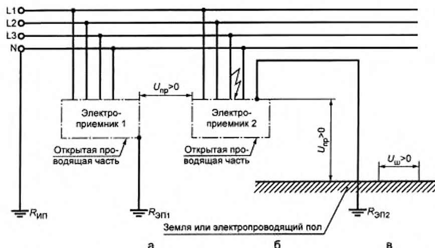
Рисунок В.10 — Сеть TT с нулевым рабочим проводником с однофазным замыканием на корпус
