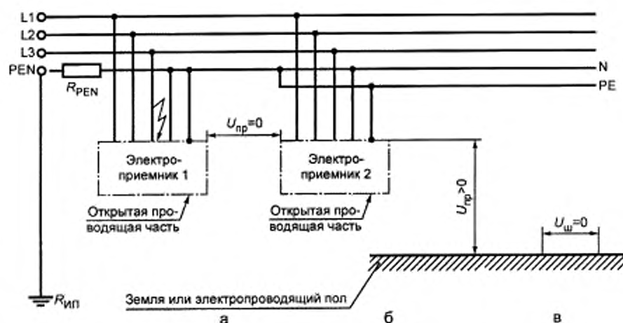
Рисунок В.9 — Сеть TN-C-S с однофазным замыканием на корпус до точки разделения PEN-проводника на N- и PE-проводники
