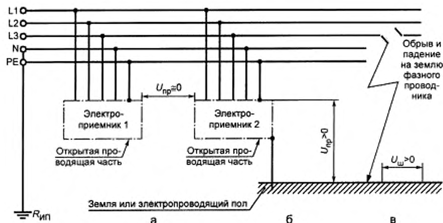
Рисунок В.5 — Сеть TN-S с замыканием на землю, например с оборванным и упавшим на землю фазным проводом
