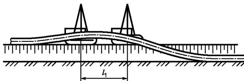
l_1 — расстояние между трубоукладчиками
