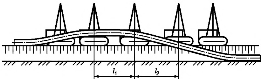
l_1, l_2 — расстояния между трубоукладчиками
