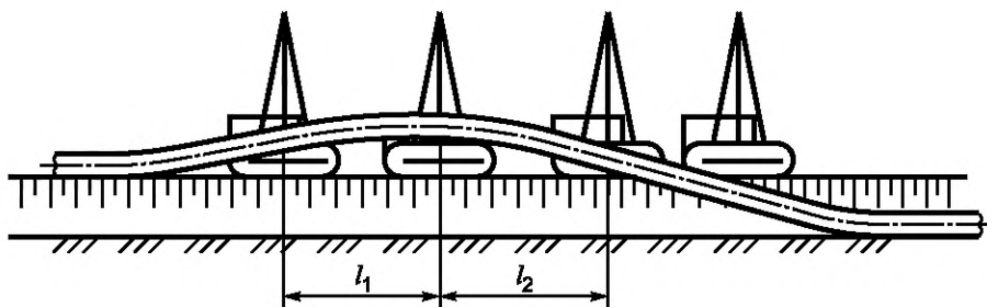
l_1, l_2 — расстояния между трубоукладчиками
