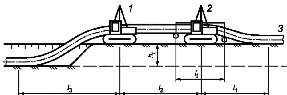
1 — задний трубоукладчик; 2 — головной трубоукладчик; 3 — трубная плет; l_1 — расстояние от начала подъема трубы до трубоукладчика; l_2 — расстояние между трубоукладчиками; l_3 — расстояние от трубоукладчика до конца опуска трубы в траншею; h_t — глубина траншеи; l_t — расстояние между опорными точками траверсы трубоукладчика
