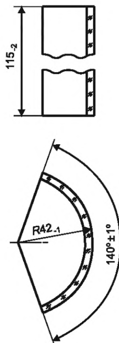
Рисунок 1 — Светофильтр цилиндрический
