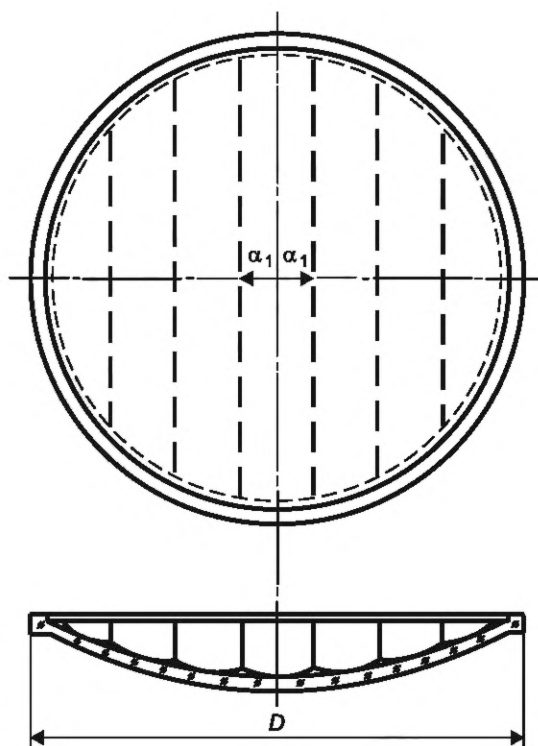
Рисунок 8 — Двухсторонний рассеиватель
