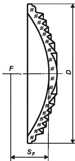
Рисунок 5 — Светофильтр-линза СЛ 139
