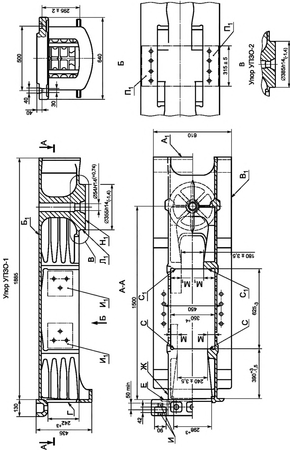
Рисунок 14 — Упоры передний и задний объединенные УПО-1, УПО-2
