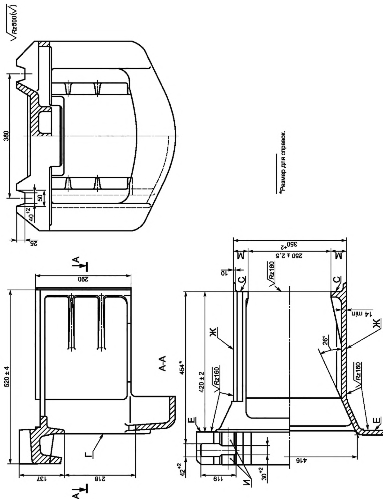
Рисунок 7 — Упор передний УПЗ-2
