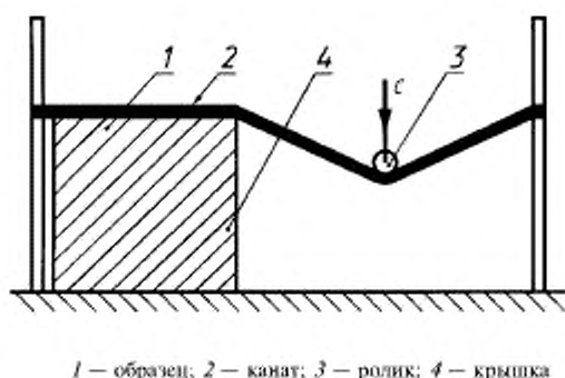
1 — образец; 2 — канат; 3 — ролик; 4 — крышка
