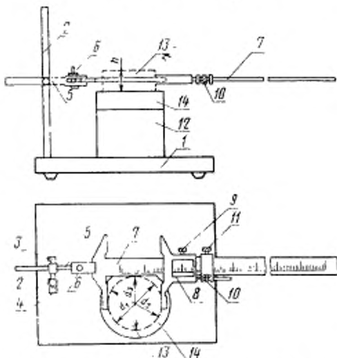
1—основание; 2—стойка; 3—стопор горизонтального перемещения держателя; 4—стопор вертикального перемещения держателя; 5—держатель штангенциркуля; 6—крепежный винт; 7—штангенциркуль с погрешностью измерения 0,05 мм; 8—ноннус; 9—стопор ноннуса; 10—микрометрический винт; 11—стопор микрометрического механизма; 12—подкладка; 13—образец грунта; 14—предметный столик.
