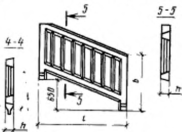
Панель ограждения лестничного марша
