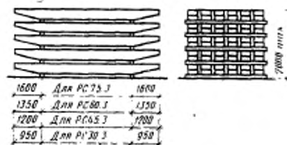
Стойки и свая-стойки
