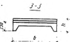
Панель ограждения лестничного марша
