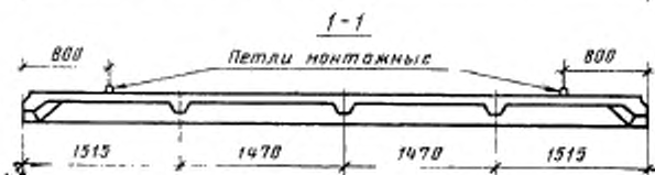
Лестничный марш
