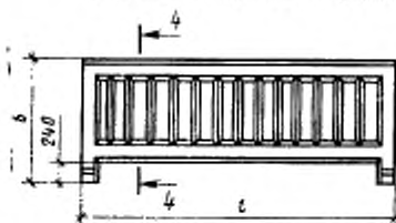
Панель ограждения платформы
