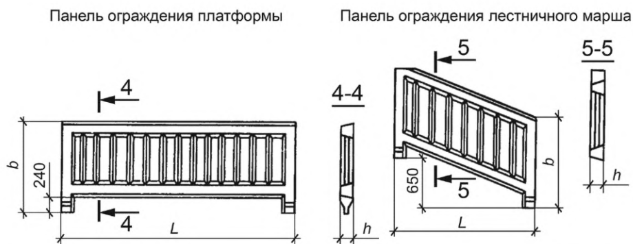
Рисунок 1 — Форма и размеры плит и лестничных маршей
