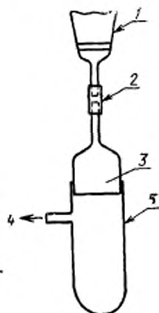
Фильтровальная пробирка для фильтрации экстракта
