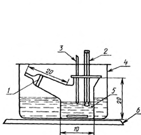
Установка для экстрагирования с фильтровальным стаканом
