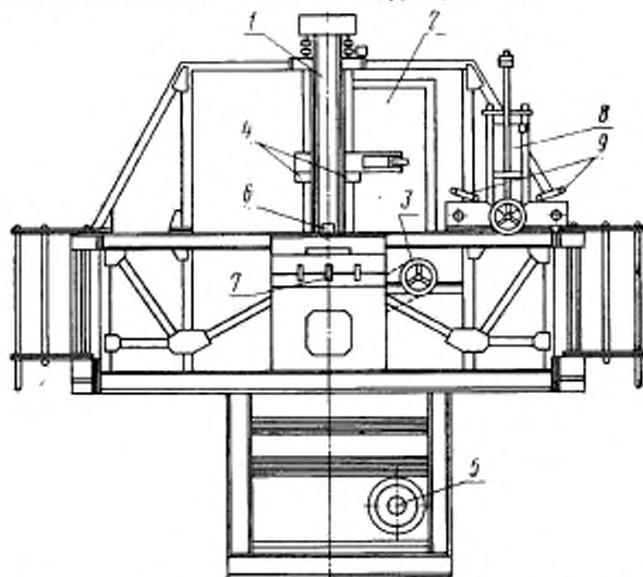
1—стойка; 2—испытуемое изделие; 3—привод; 4—рычаги-толкатели; 5—гидробак; 6—счетчик оборотов; 7—пульт управления; 8—нагружающее устройство; 9—стойловое устройство.
