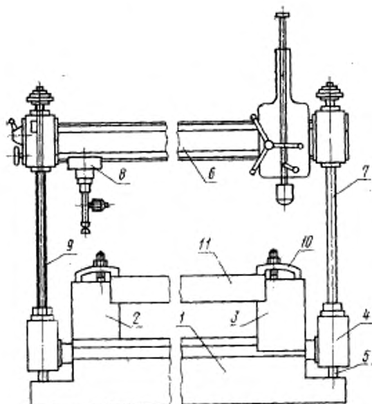
1—основание машины; 2—неподвижная опора; 3—подвижная опора; 4—каретка; 5—направляющая каретки; 6—трaverse; 7—ходовка для перемещения traverse; 8—датчик сил; 9—измеритель перемещений; 10—прижимы; 11—испытуемое изделие.
