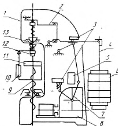
Схема прибора ПСП-80
