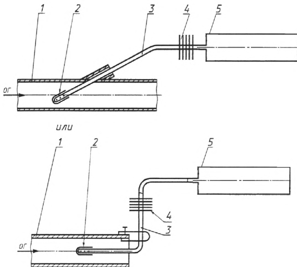
1 - прямолинейный участок выпускной трубы двигателя; 2 - газоотборный зонд; 3 - линия отбора; 4 - охладитель; 5 - дымомер.
