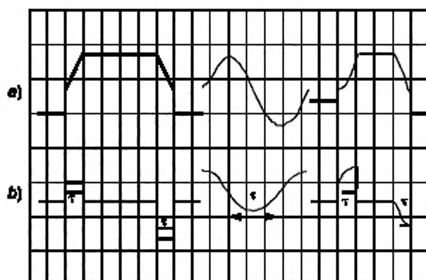
а) Возможные законы изменения во времени градиентного магнитного поля. б) Скорость изменения во времени градиентного магнитного поля dB/dt .
