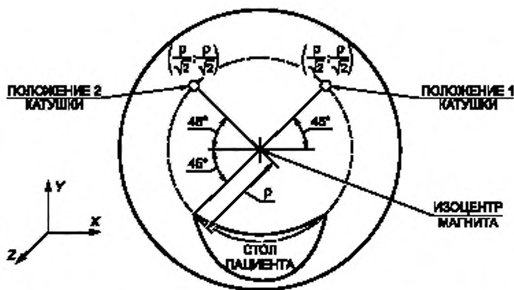
Рисунок 103 — Положения измерительной катушки при измерениях \frac{dB}{dt}
