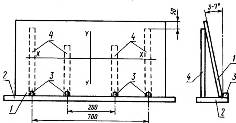
Схема стенда с установленным образцом
