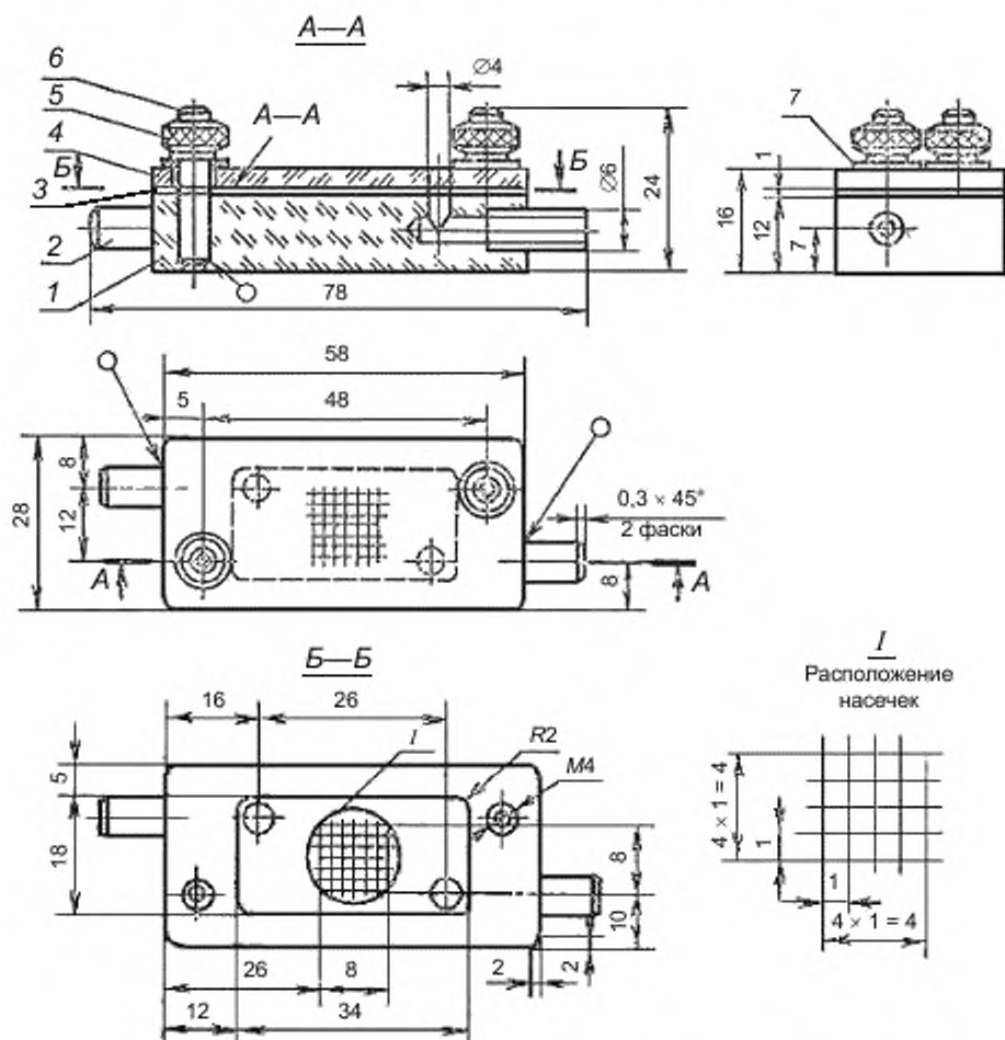
1 — основание; 2 — патрубки; 3 — прокладка; 4 — крышка; 5 — гайка; 6 — шпильки; 7 — шайбы
