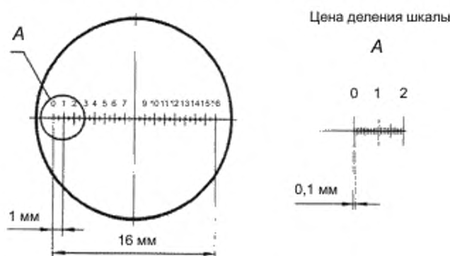
Рисунок 2 — Линейный окуляр-микрометр
