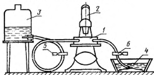
1—счетная камера; 2—микроскоп; 3—склянка; 4—емкость; 5, 6—зажимы
