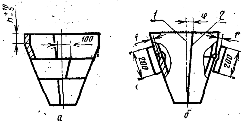
1—образующая; 2—продольный шов.
