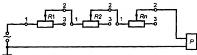
R1, R2, \dots Rn — проверяемые резисторы; 1, 2, 3 — выводы проверяемых резисторов; P — осциллограф
