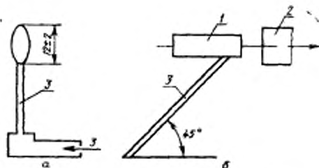
a —положение газовой горелки при установке высоты пламени, б —то же, во время испытания резистора; 1—испытываемый резистор; 2—приспособление для крепления испытываемого резистора; 3—газовая горелка
