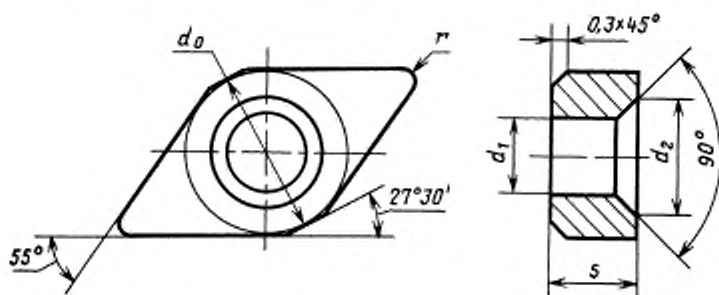
Размеры, мм
