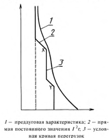
Рисунок 1 — Пример условной кривой перегрузок (X и Y — точки, для которых проверяется стойкость против перегрузок)
