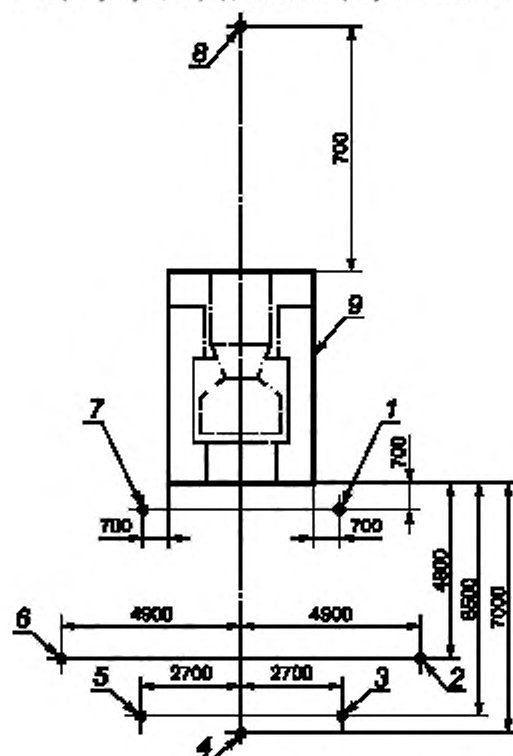
1—8 — точки измерений уровней звука, 9 — прямоугольный параллелепипед, описанный вокруг трактора (без навесного оборудования)
