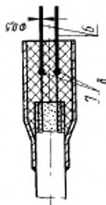
Выводы термоэлектродов для кабельных термопреобразователей диаметрами 1,0 и 1,5 мм
