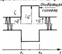
Форма сигнала на входе усилителя
