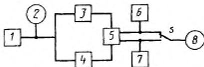
1 — генератор; 2, 8 — вольтметры; 3, 4 — эквиваленты полного сопротивления источника; 5 — измеряемый усилитель; 6, 7 — эквиваленты нагрузки; 8 — переключатель
