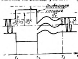
Форма сигнала на выходе усилителя (пример)
