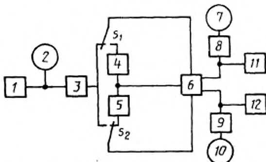
1 — генератор; 2, 7, 10 — вольтметры; 3 — согласующее звено; 4, 5 — эквиваленты сопротивления источника; 6 — измерительный усилитель; 8, 9 — фильтры; 11, 12 — эквиваленты нагрузки; S_1 , S_2 — переключатели
