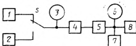
1 — генератор высокого тона; 2 — генератор; 3, 6 — вольтметры; 4 — согласующее звено; 5 — измеримый усилитель; 7 — самописец; 8 — эквивалент нагрузки; 5 — переключатель
