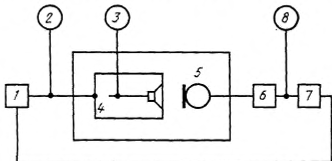
1—УАЗЧ; 2, 3, 8—электронный вольтметр; 4—испытуемое изделие; 5—измерительный микрофон; 6—усилитель УМ; 7—следящий анализатор спектра
