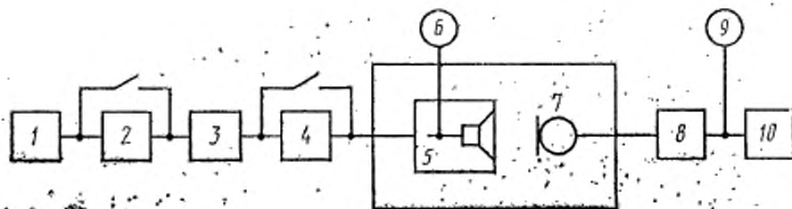
1 — генератор ГНИ; 2 — стереофонический модулятор; 3 — генератор ГСВ2; 4 — эквивалент антенны; 5 — испытуемый радиовещательный приемник; 6, 9 — электронный вольтметр; 7 — измерительный микрофон; 8 — усилитель УМ; 10 — ИНИ, анализатор спектра или селективный вольтметр
