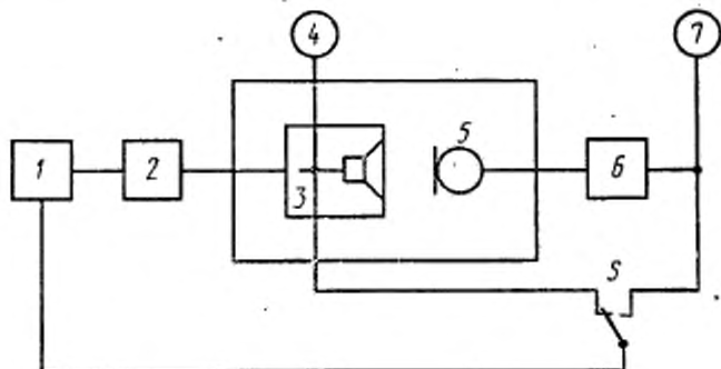
1 — ГНИ с регистрирующим устройством; 2 — ГСВ1; 3 — испытуемый трехпрограммный приемник; 4, 7 — электронный вольтметр; 5 — измерительный микрофон; 6 — усилитель УМ; S — переключатель
