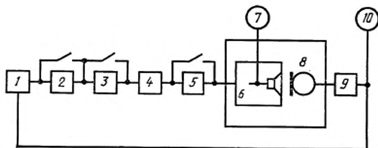
1—УАЗЧХ; 2—цель предискажений; 3—стереофонический модулятор; 4—генератор ГСВ2; 5—эквивалент антенны; 6—испытываемый радиовещательный приемник; 7, 10—электронный вольтметр; 8—измерительный микрофон; 9—усилитель УМ
