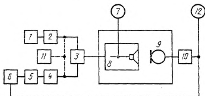
1—генератор полного телевизионного сигнала; 2—генератор ГСВ1; 3—разветвитель; 4—генератор ГСВ2; 5—цель предискажений; 6—УАЗЧХ; 7, 12—электронный вольтметр; 8—испытываемый телевизионный приемник; 9—измерительный микрофон; 10—усилитель УМ; 11—электронно-счетный частотомер
