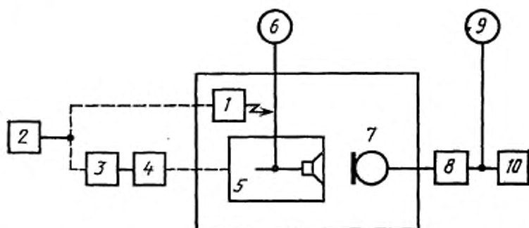
1—генератор поля; 2—генератор ГНИ; 3—генератор ГСВІ; 4—эквивалент антенны; 5—измеряемый радиовещательный приемник; 6, 9—электронный вольтметр; 7—измерительный микрофон; 8—усилитель УМ; 10—ИНИ, анализатор спектра или селективный вольтметр
