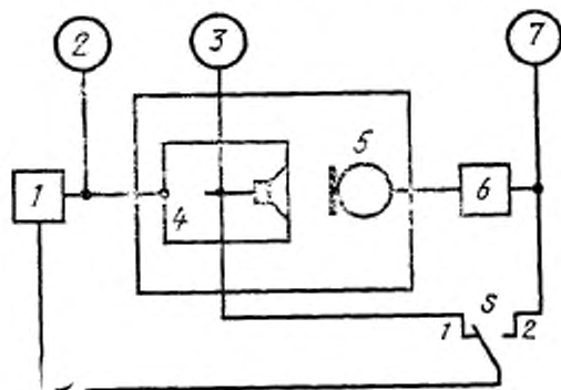
1—УАЗЧХ; 2, 3, 7—электронный вольтметр; 4—испытываемое изделие; 5—направительный микрофон; 6—усилитель УМ; S—переключатель
