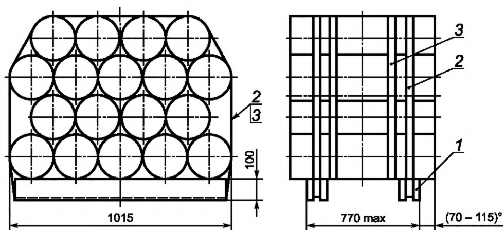
Рисунок А.2 — Схема упаковки короткомерных слитков в горизонтальные пакеты
