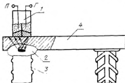
1 — раздельно совмещенные искатели; 2 — сварное соединение; 3 — стержень; 4 — пластина закладной детали, I — вывод к генератору ультразвуковых колебаний, II — вывод к приемнику.
