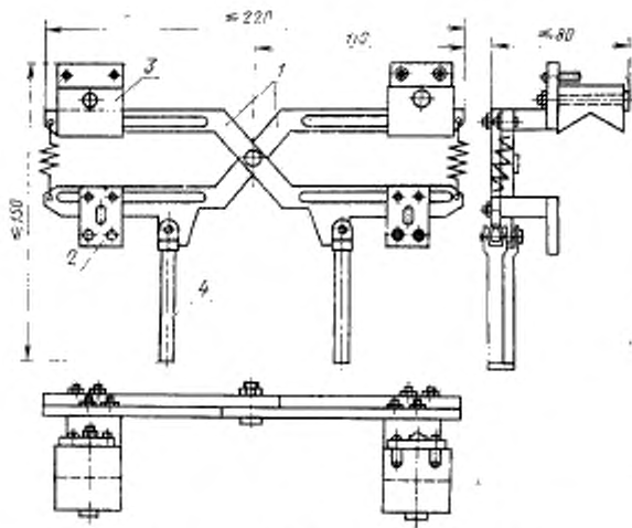
1 — рычаги; 2 — планка крепления искателя; 3 — фиксатор; 4 — рукоятка.
