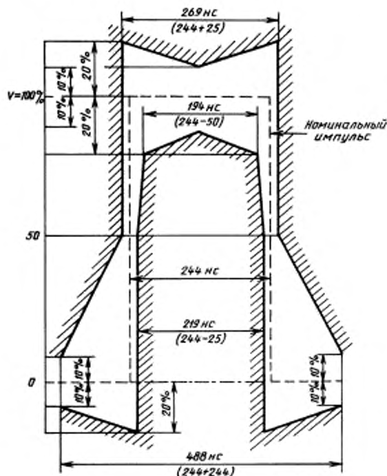
Вид и форма импульса кодированного сигнала
