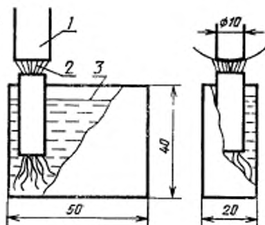
1 — контробразец; 2 — фитиль; 3 — масло
