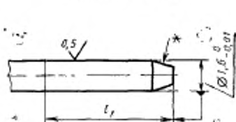
Хвостовик типа 3
