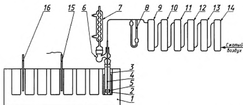
1 — термостат; 2 — стакан алюминиевый; 3 — реактор; 4 — трубка подачи воздуха; 5 — пластины металлические; 6 — приемник конденсата; 7 — конденсатор; 8 — реометр; 9 — колонка с ватой; 10 — колонка с аскаритом; 11 — колонка с силикагелем-индикатором; 12 — колонка с мелкопористым силикагелем; 13 — колонка с крупнопористым силикагелем; 14 — колонка с хлористым кальцием; 15 — термометр; 16 — термостат; 17 — крышка
