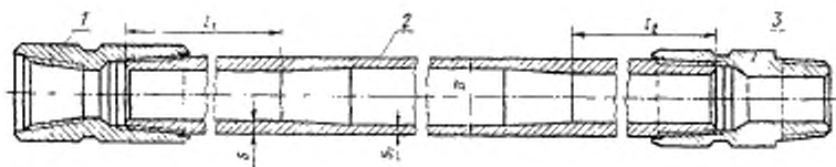
1—муфта замка; 2—труба; 3—гайка замка
