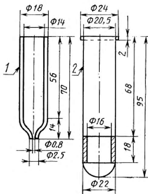
Центрифужная пробирка и оболочка
