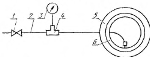
1—вентиль; 2—трубопровод; 3—манометр; 4—тройник; 5—шина; 6—обод
