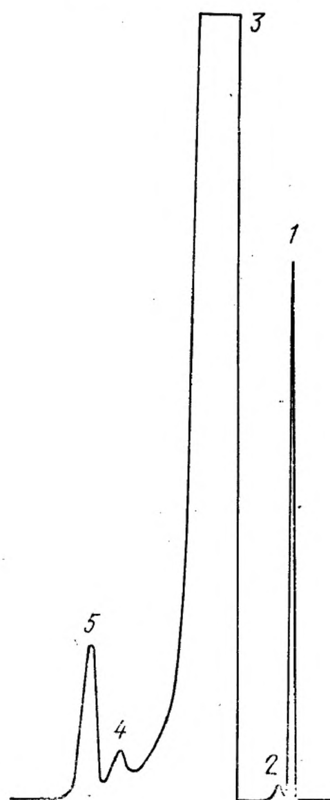
Типовая хроматограмма товарного хладона 113
