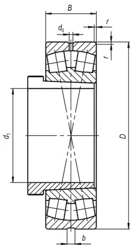
Рисунок 7 — Конструктивное исполнение 07Н
