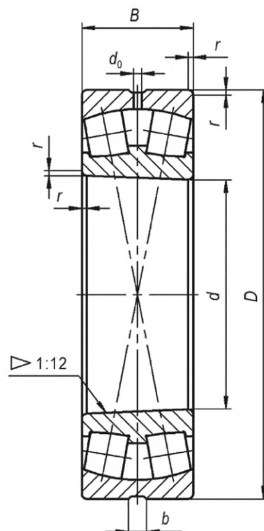
Рисунок 10 — Конструктивное исполнение 11Н, серии ширин 0 и 3
