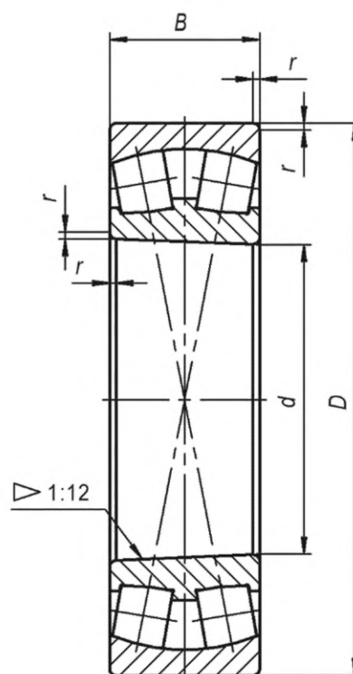
Рисунок 8 — Конструктивное исполнение 11, серии ширин 0 и 3
