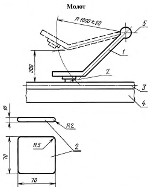
1 — молот; 2 — ланка; 3 — ампульпровод; 4 — горизонтальная плита массой 150 кг; 5 — горизонтальная ось
