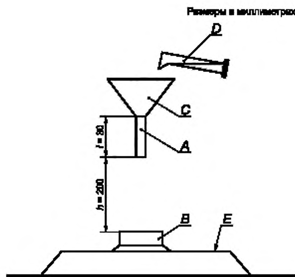
А — воронка с трубкой, внутренний диаметр которой составляет 8 мм; В — испытуемый предмет; С — воронка; D — контейнер с 30 мл соляного раствора; E — горизонтальная поверхность
