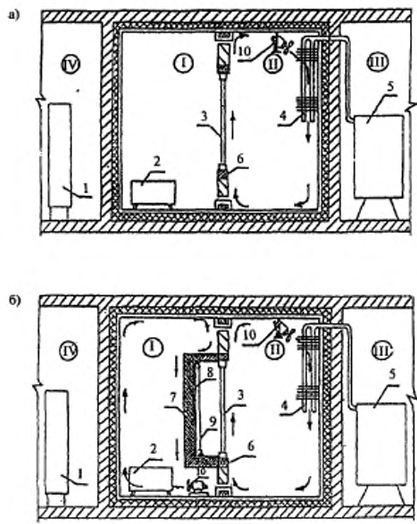
I — теплое отделение камеры; II — холодное отделение камеры; III — машинный зал; IV — помещение с измерительной аппаратурой; 1 — система автоматического сбора данных; 2 — нагревательные приборы; 3 — испытываемый оконный блок; 4 — испаритель; 5 — холодильная установка; 6 — теплоизоляционный слой по периметру проема; 7 — калориметр (утепленная приставная камера); 8 — металлическое отражающее покрытие; 9 — спираль нагрева, равномерно распределенная по площади калориметра; 10 — вентилятор
