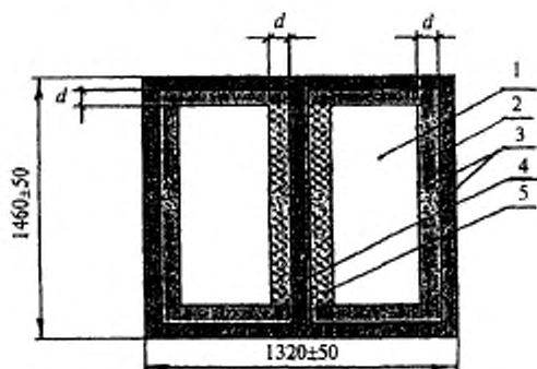
1 — центральная зона остекления; 2 — краевая зона остекления; 3 — коробка и створка; 4 — разделительная деталь (импост); 5 — краевая зона остекления у разделительной детали
