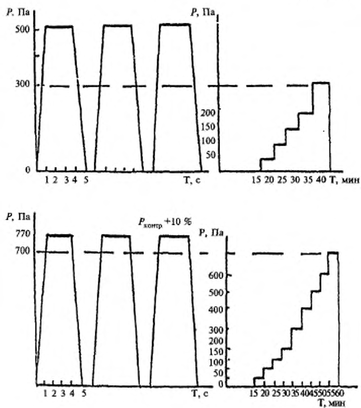
Рисунок 5 — Примеры построения графиков испытаний оконных блоков на водонепроницаемость для конечного контрольного давления 300 и 700 Па
