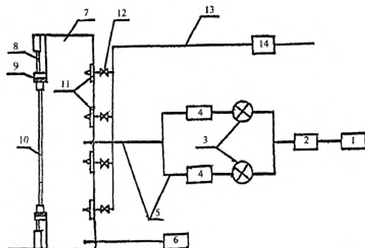
1 — компрессор (воздушный насос); 2 — регулятор расхода воздуха; 3 — воздушные запорные краны; 4 — ротаметры с различными пределами измерения; 5 — шланги; 6 — датчик давления (манометр); 7 — герметичная камера; 8 — приспособление для крепления образца; 9 — эластичные уплотнительные прокладки; 10 — образец. Дождевальное оборудование: 11 — форсунки; 12 — запорные устройства (вентили). 13 — шланг для подачи воды; 14 — счетчик воды
