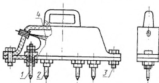
Схема четырехзондового датчика
