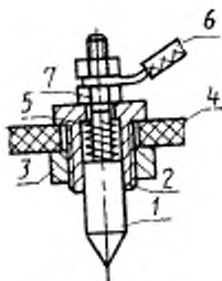
Схема зонда
