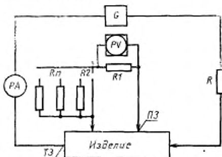
G — источник постоянного тока; PA — прибор для измерения тока; PV — прибор для измерения напряжения; R — ограничивающий резистор; R1—Rn — резисторы делителя напряжения; TZ — токовый зонд; ПЗ — потенциальный зонд.
