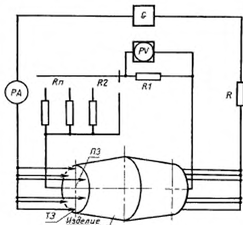
G — источник постоянного тока; РА — прибор для измерения тока, РV — прибор для измерения напряжения, R — ограничивающий резистор; R1—Rn — резисторы делителя напряжения; ТЗ — токовый зонд; ПЗ — потенциальный зонд
