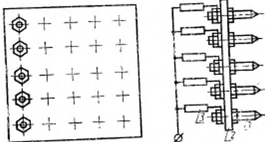
Схема датчиков токовых зондов
