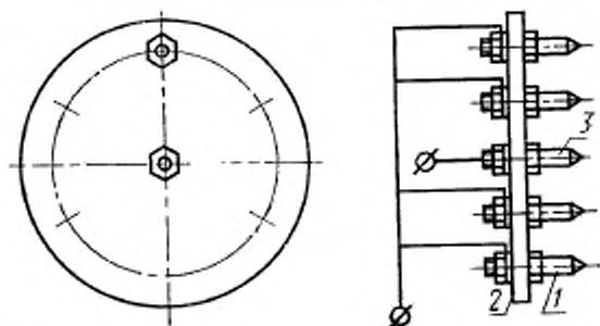
Схема комбинированного датчика
